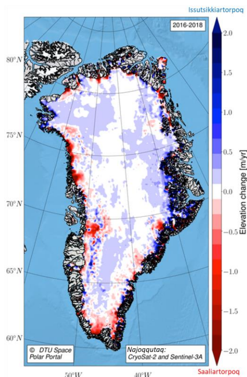
Takuss. 7: Nunap assingani piffissami januar 2016-imiit december 2018-imut ukiut tamaasa qatsissutsit allanngorneri takuneqarsinnaapput nalunaarsuutit Sentinel-3A aamma CryoSat-2-meersut najoqqutaralugit.
