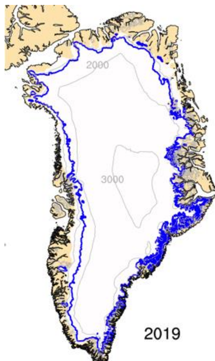
Takuss. 3: Nunap assingata takutippaa aaffiup nalaata naanerani aputip killinga sumiinnersoq, t.i. qatsinnerusumi aputaavoq atsinnerusumilu sermiulluni. Titarnerup takutippaa sermeqarfiusoq qanoq annertutiginsorq. 2019-imi sermeqarfiusoq maangamut uuttorneqarsimasoq anginerpaavoq, 2012-iminngarnit anginerulaaginnarluni.
