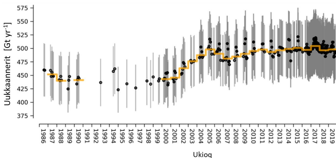
Takuss. 6: Uukkaannerit piffissanut nalunaarsorneri. Toornerit alapernaarsuinerit qanga piskasut nalunaarpaat (killiliissut > 50%-imik inunngisaa). Titarnerup orangeap kipisimasup agguaqatigiissut ukiumoortoq takutippaa (ukiumut alapernaarsuinerit 3-innaapput imaluunniit 4-annaapput).
