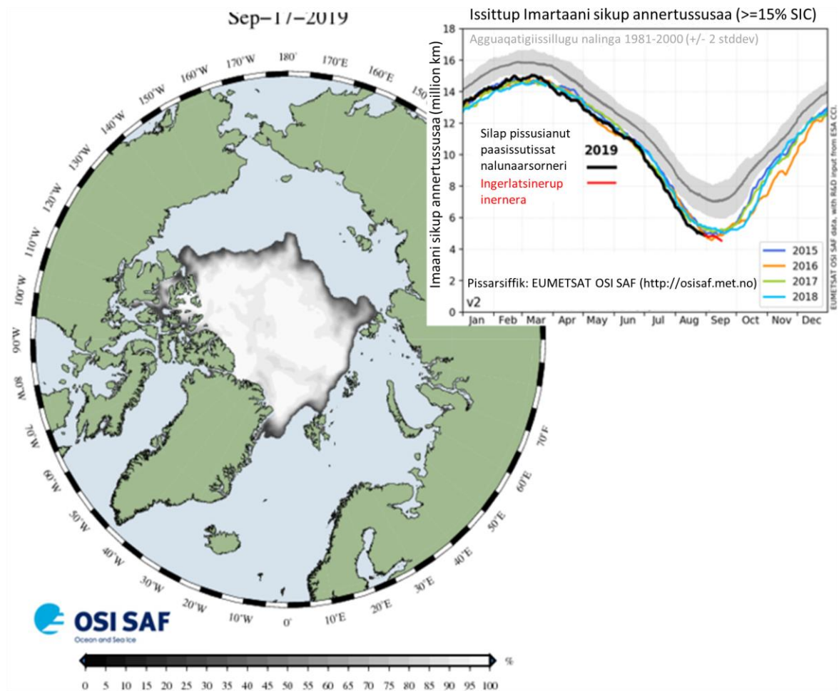
Takuss. 9: Immap sikuata siammarsimassusia pillugu DMI’p titarnera 17. september 2019-imeersoq, ukiup naatsorsuiffiusup ullua sikup annikinnerpaamik siammarsimassusia. Nunap assinga aamma titartagartaliussineq EUMETSAT’s OSISAF’ip sikut eqimassusii pillugit naatsorsuinerannik tunngaveqarpoq, takutillugulu imartat 15%-imik anginerusumik sikusimasut arealii. Titartagartaliussaq Polar Portalimiit.
