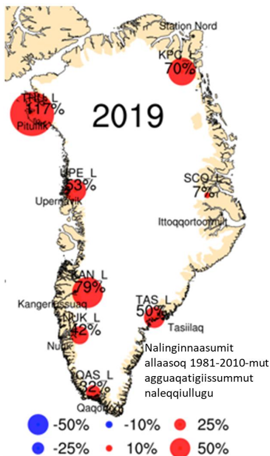
Takuss. 4: Nunap assingisa takutippaat silasiorfinni PROMICE-ni atsinnerusumiittuni 2019-imut ilanngaattissat ilanngaatigereerlugit aassimasup nikinganeri (nalinginnaasumit allaasoq) piffissanut 1981-2010 (saamerleq) aamma 2011-2015 (talerpilleq) naleqqiullugit.
