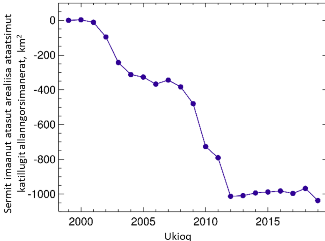
Takuss. 5: Titarnerup ersersippaa Kalaallit Nunaanni sermit imaanut atasut anginerpaat 7 arealiisa ataatsimut katillugit allanngorsimanerat. Takutippaa sermit taakku 2018-imiilli areali -71,2 \pm 1,4 \text{ km}^2 annaasimagaat. Taamatut annaasaqarneq ukiuni 2013-2018 aalaakkaakannersumik annertuumik annaasaqarfiusimanngitsup kingorna annaasaqarfiuvoq annerpaaq.
