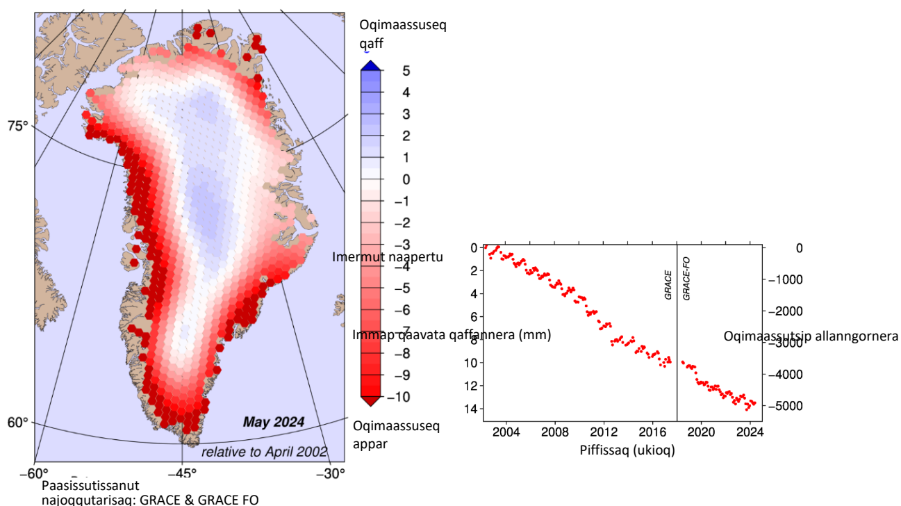
Assitaliussaq 5: Grafimi takutinneqarput sersersuup ataatsimut annertussusaata qaammatikkaartumik allannguutai Gt-inngorlugit, GRACE-mit aamma GRACE-FO-mit paasisutissat tunngavigalugit. (1 Gt-ip assingaa 1 mia. ton imaluunniit imeq 1 km 3 . 100 Gt-ip assingaa nunarsuup tamarmi imartaasa 0,28 mm-imik qaffariarnerat). GRACE qullartinneqarpoq 2002-mi martsimi, uuttortaaneralu naammassivoq 2017-imi oktoberimi. GRACE-FO qullartinneqarpoq 2018-imi majimi, taamaammat qaammataasiat marluk taakku akornanni paasisutissat amingarput. Paasisutissat kingulliit 2024-mi majimeersuupput (Tunngavik: Polarportal).
