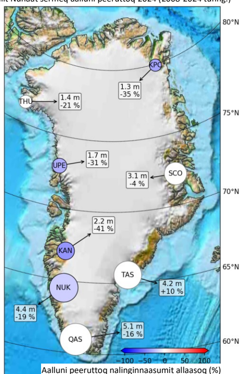
Kalaallit Nunaat sermeq aalluni peeruttoq 2024 (2008-2024 tunng.)
