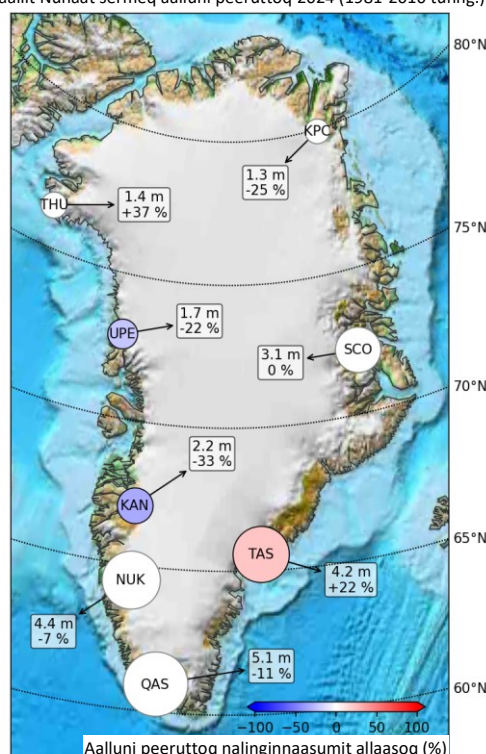
Kalaallit Nunaat sermeq aalluni peeruttoq 2024 (1981-2010 tunng.)
